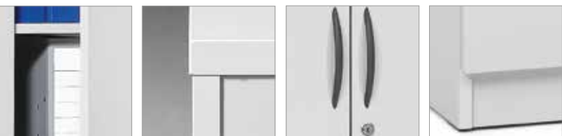
Holzfachböden 18 mm stark Sichrückwände , 12 mm stark Ergonomische Griffe aus Metall, Zylinderschloss mit 2 Schlüsseln Sockel mit Bodenausgleich, von innen einstellbar
